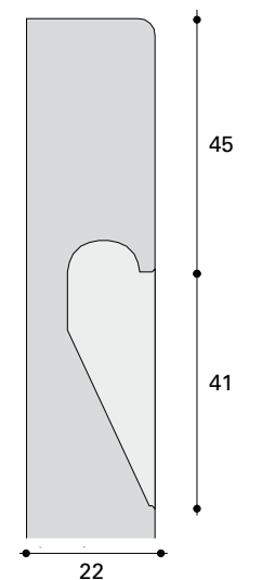
Sezione anta Door section
