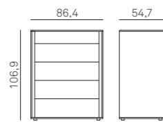
Elemento 5 cassetti P=54,7 H=106,9
