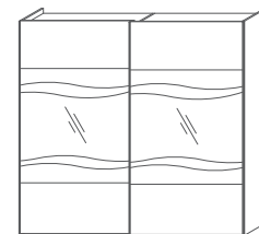
FESTIVAL (2 ante, scorrevoli) CM L.272,5xP.66x H.259
