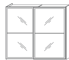
DIVA (2 ante, scorrevoli) CM L.288xP.68xH.250
