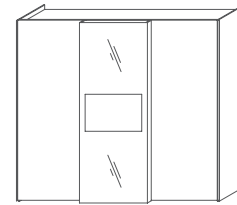
ARMADIO TV (3 ante, scorrevoli) CM L.273xP.71xH.246
